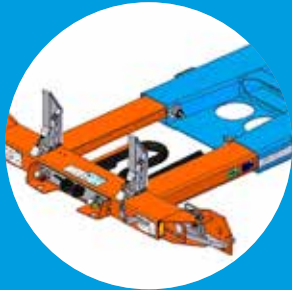
A. Flexilock (voor 45' containers)
